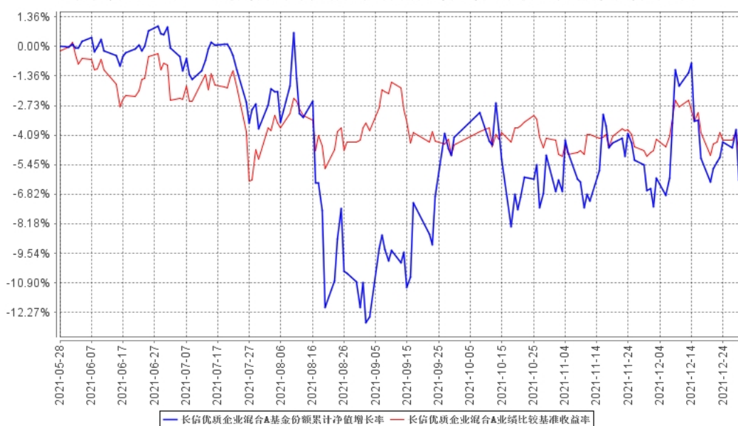
长信优质企业混合A基金份额累计净值增长率与同期业绩比较基准收益率的历史走势对比图
