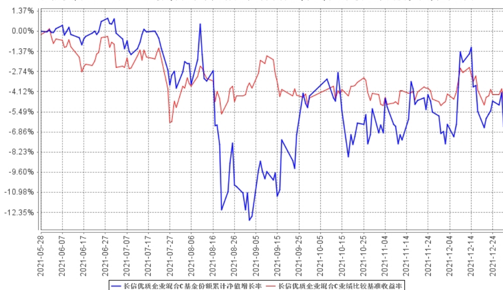
长信优质企业混合C基金份额累计净值增长率与同期业绩比较基准收益率的历史走势对比图
