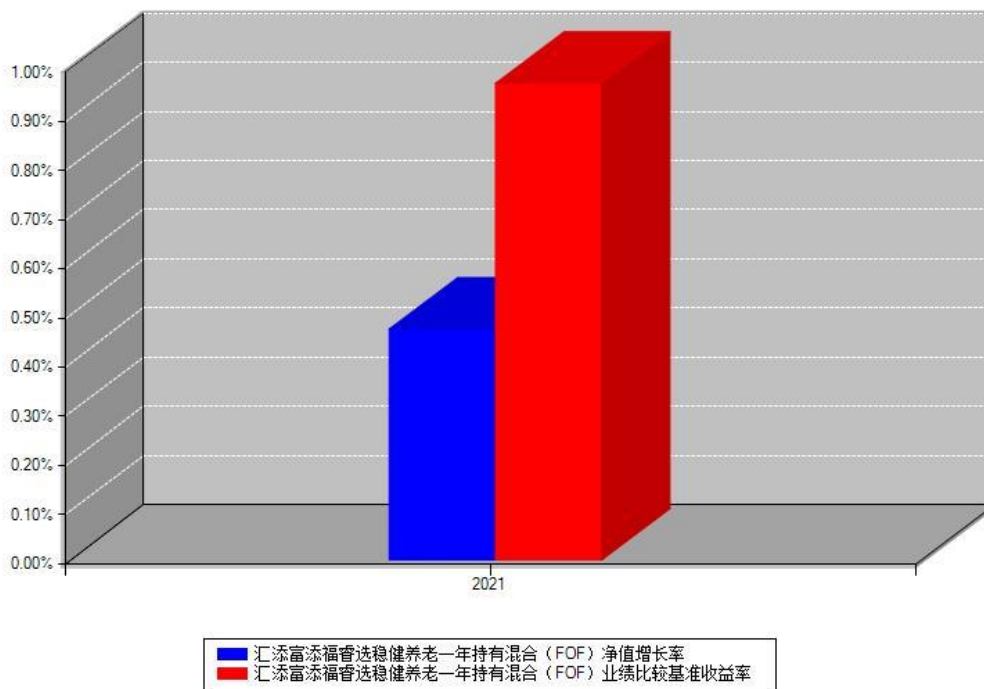
汇添富添福睿选稳健养老一年持有混合（FOF）每年净值增长率与同期业绩基准收益率对比图
