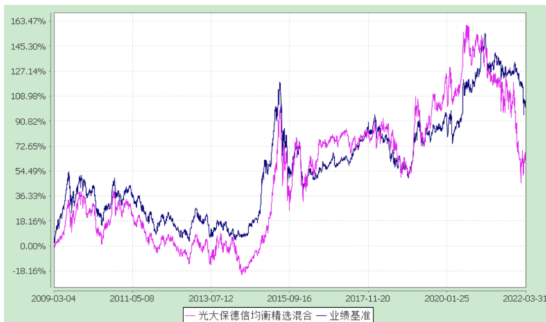
光大保德信均衡精选混合型证券投资基金 累计净值增长率与业绩比较基准收益率历史走势对比图 (2009 年 3 月 4 日至 2022 年 3 月 31 日)
