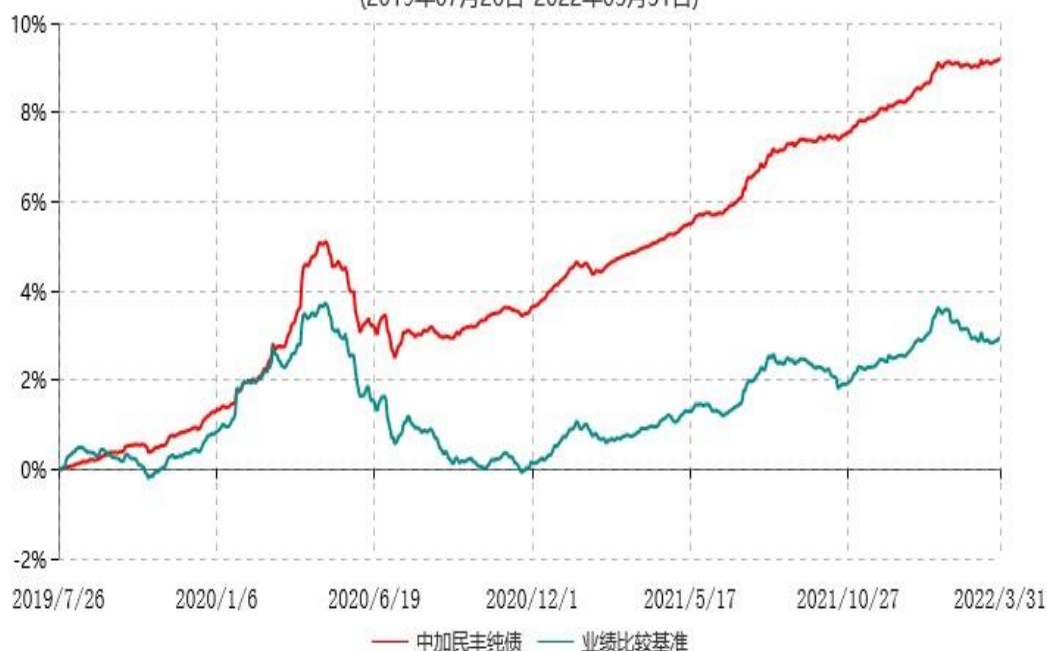
中加民丰纯债债券型证券投资基金累计净值增长率与业绩比较基准收益率历史走势对比图
