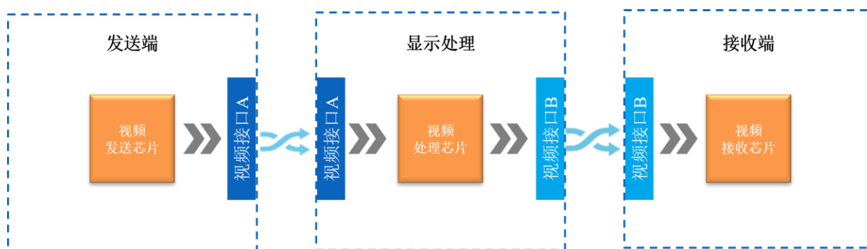
显示处理芯片应用示意图
