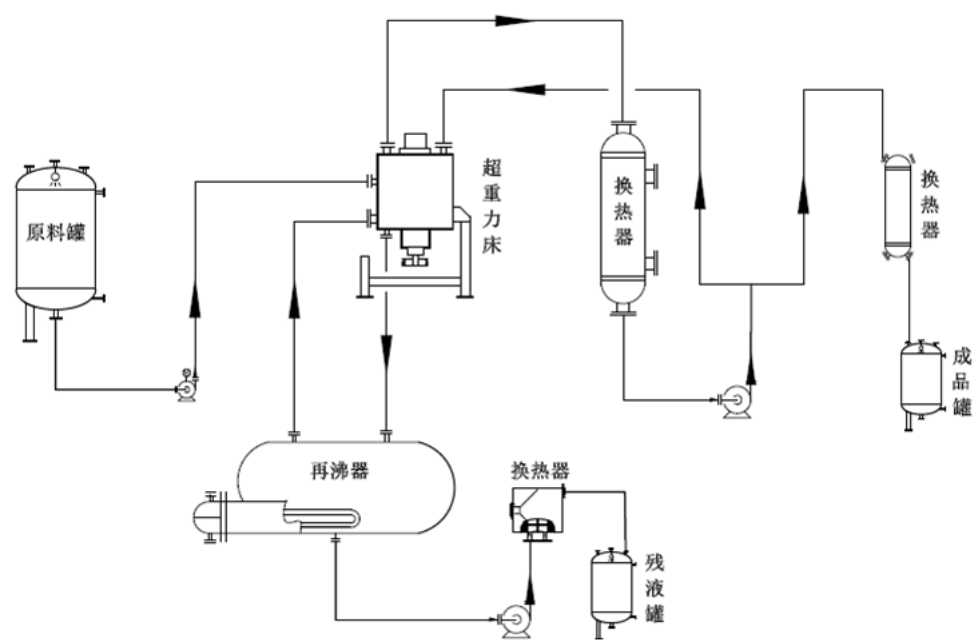
超重力精馏系统示意图
