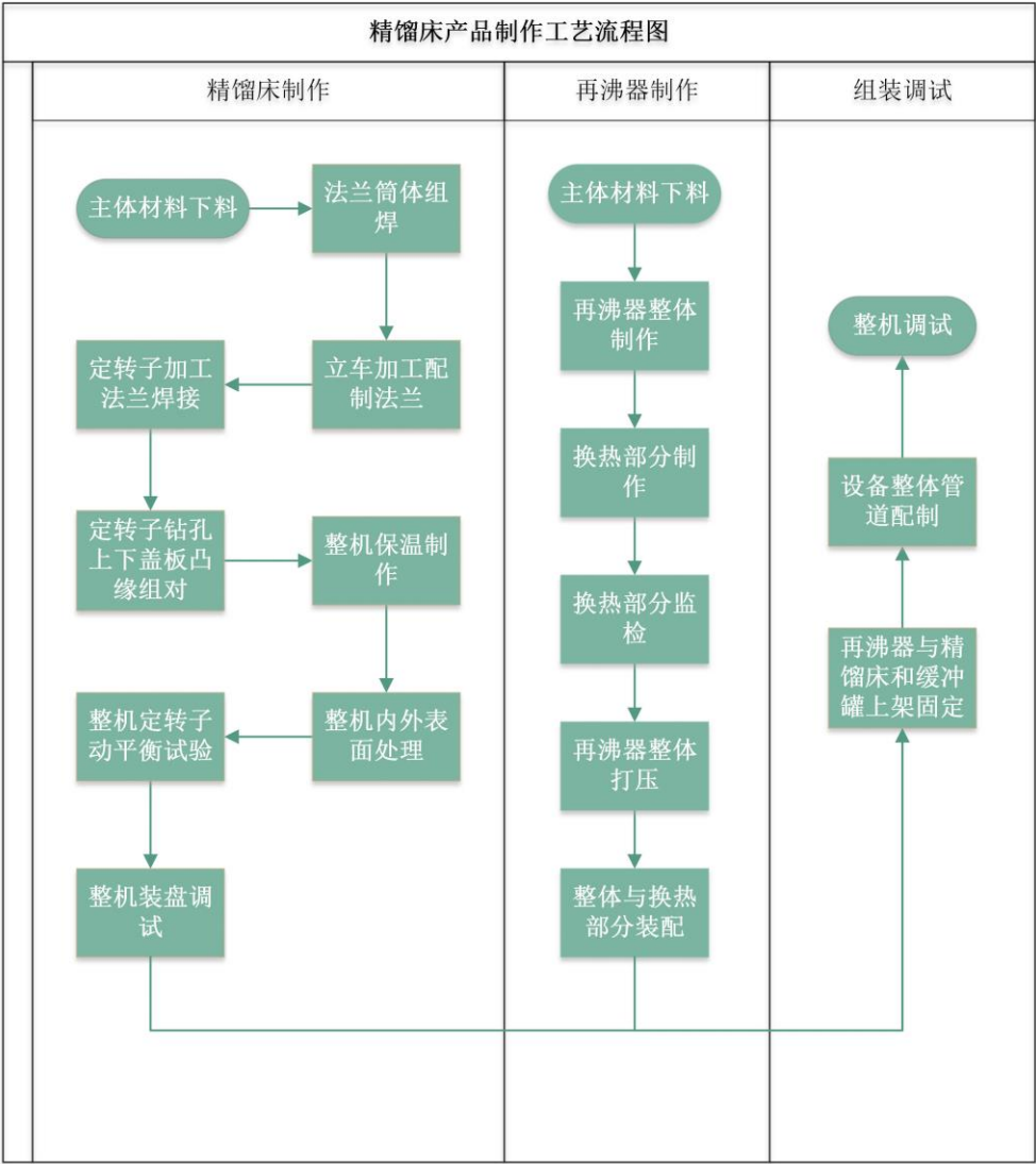
(2) 高效旋转精馏床工艺流程环节说明
