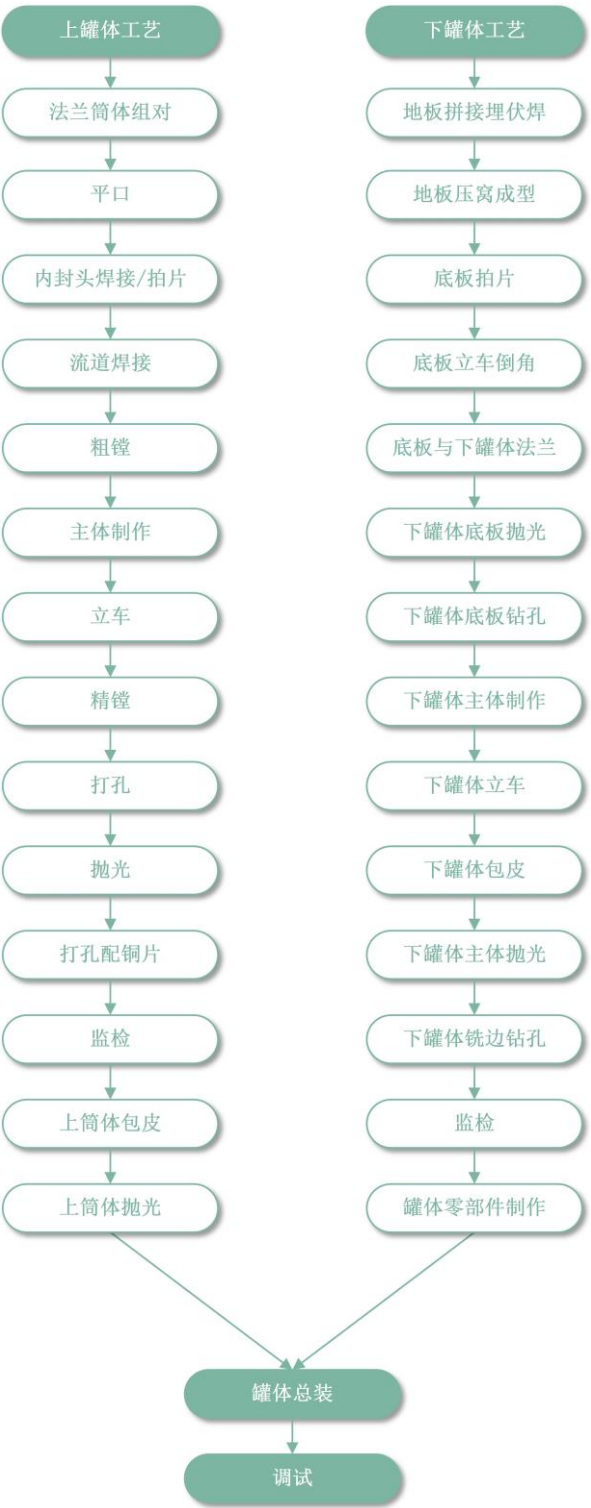
(2) 过滤洗涤干燥机工艺流程环节说明
