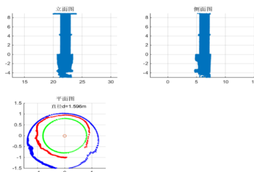
桥梁立柱病害/缺陷三视图
