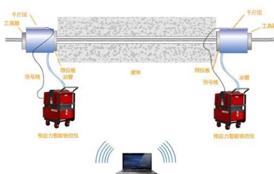
智能张拉系统原理示意图
