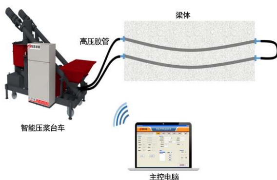
智能压浆系统原理示意图
