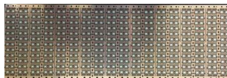
SOP 8L 的 12 排引线框架
