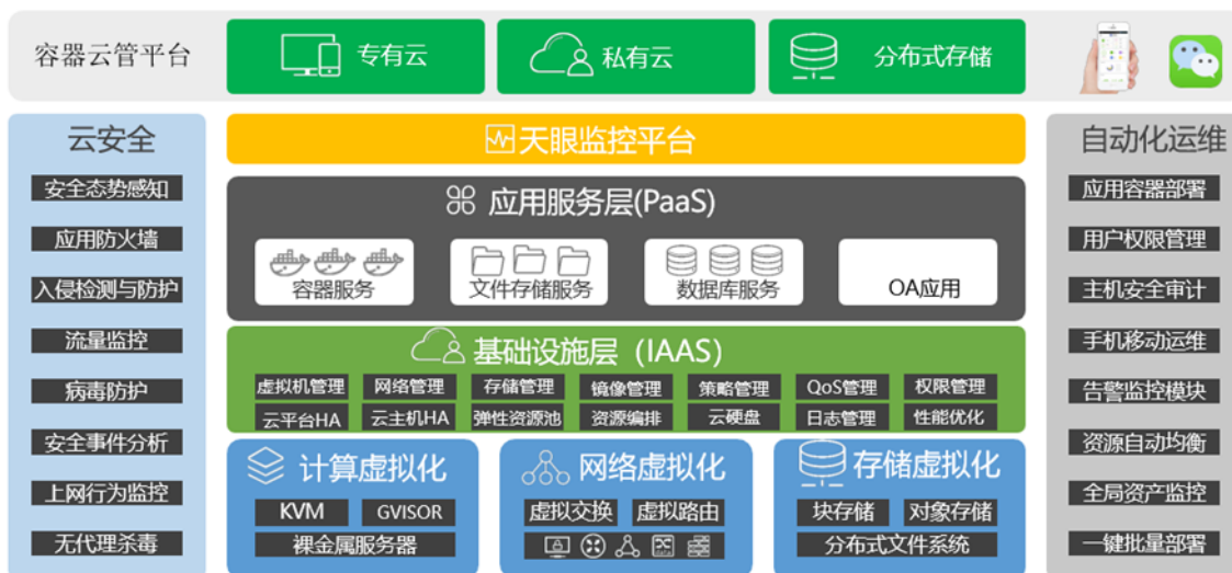
容器云管平台整体架构示意图
