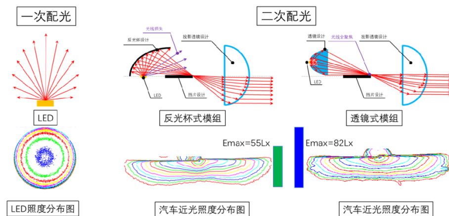
二次配光——汽车前大灯配光设计
