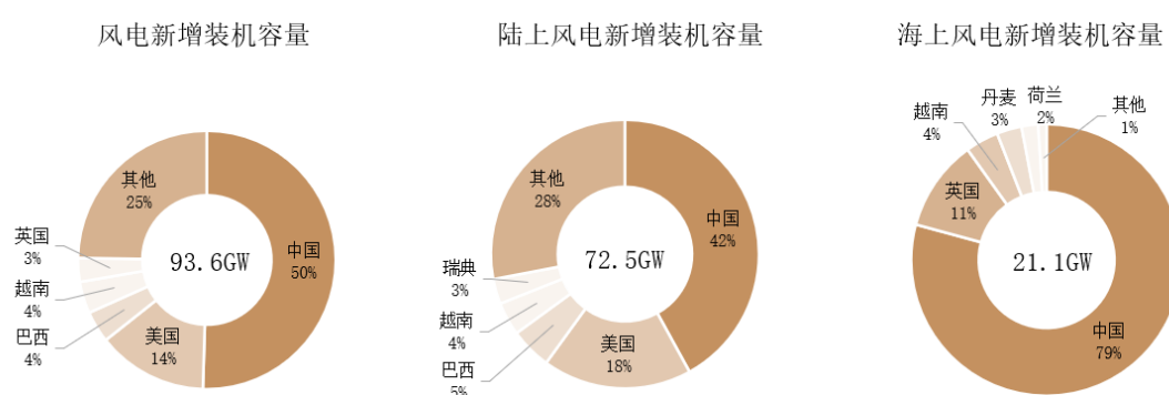
2021 年全球风电新增装机容量地域分布
