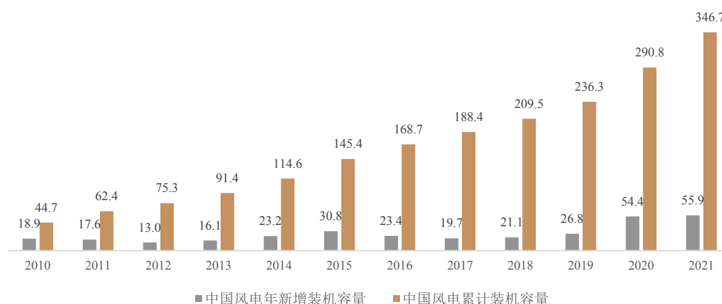
2010-2021 年我国风电累计装机容量及年新增装机容量（GW）
