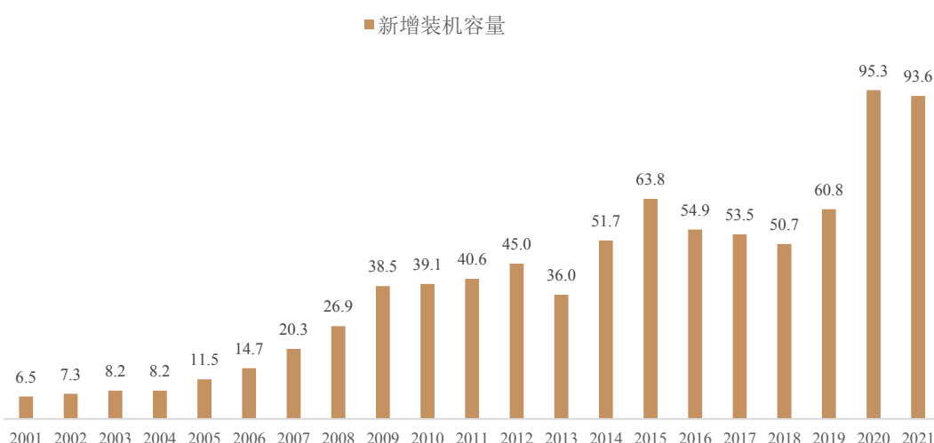
2001-2021 年全球风电新增装机容量（GW）
