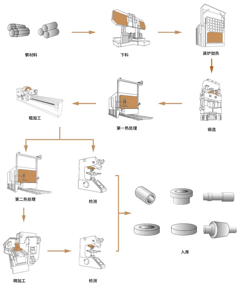
锻件工艺流程图
