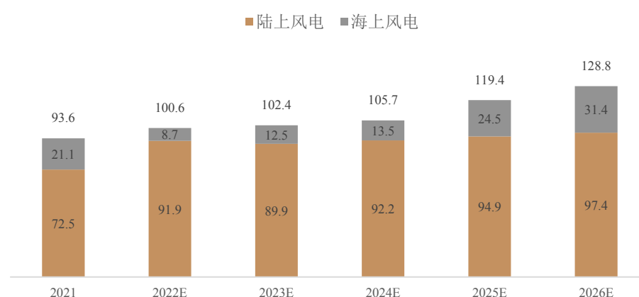
2021-2026 年全球风电新增装机容量（预测）（GW）
