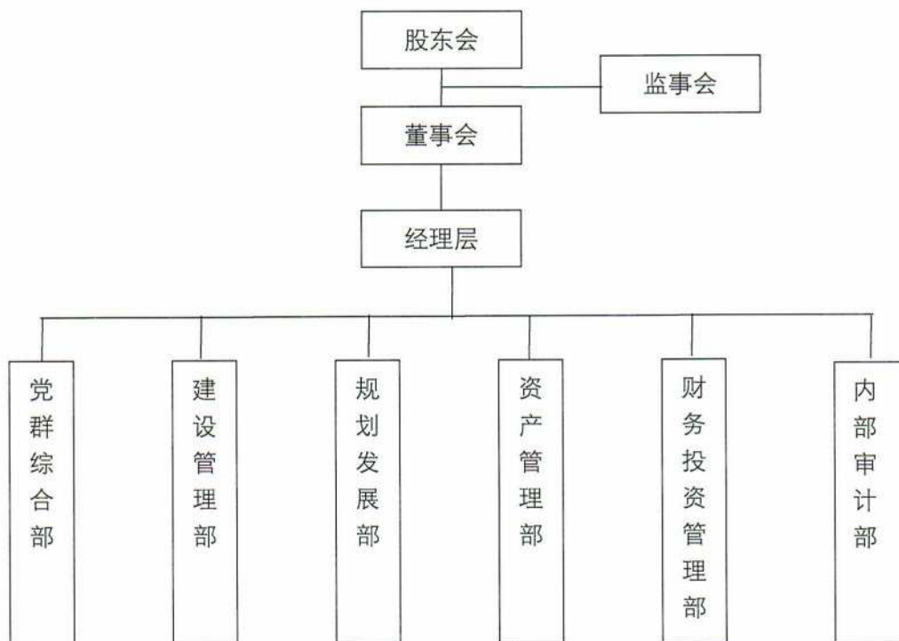
组织架构图
