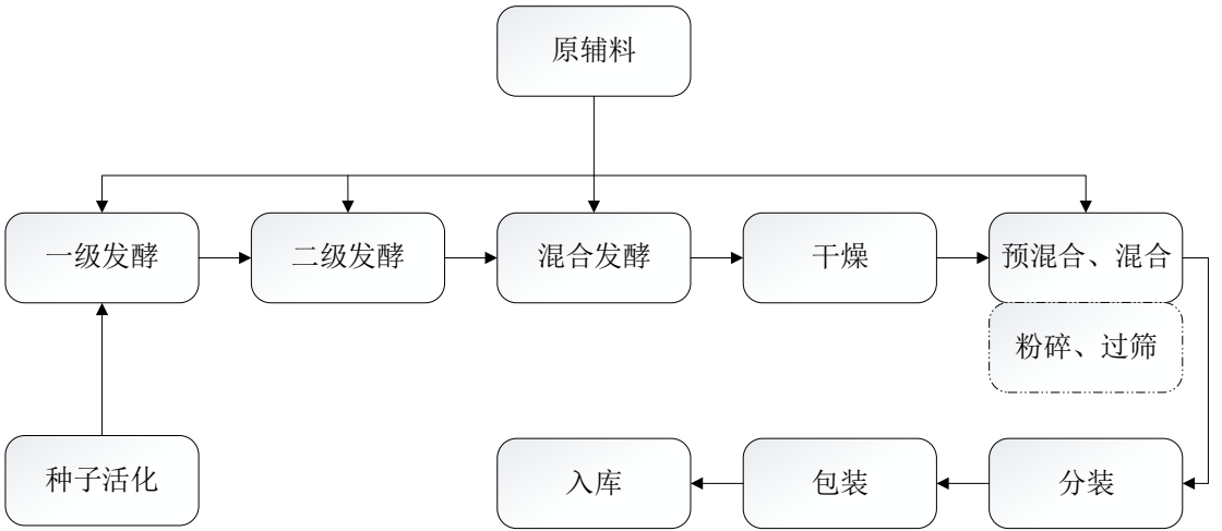
(1) 预混合饲料（固体）工艺流程图
