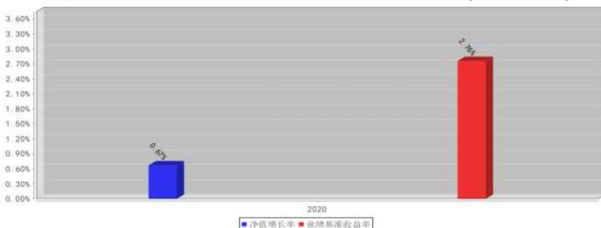
鑫元锦利定期开放基金每年净值增长率与同期业绩比较基准收益率的对比图(2020年12月31日)
