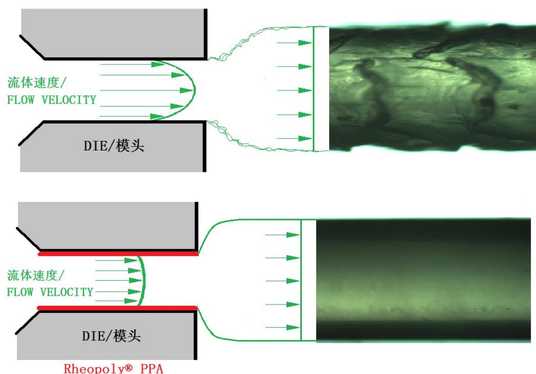
未添加的聚合物加工助剂挤出效果（上图）和添加聚合物加工助剂的挤出效果（下图）
