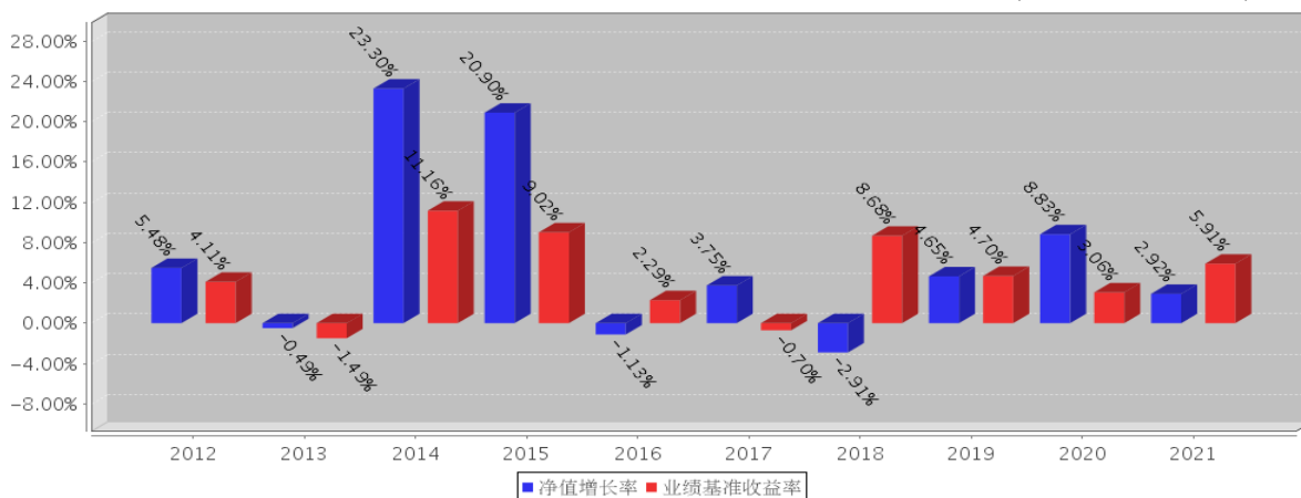
建信收益增强债券C基金每年净值增长率与同期业绩比较基准收益率的对比图(2021年12月31日)
