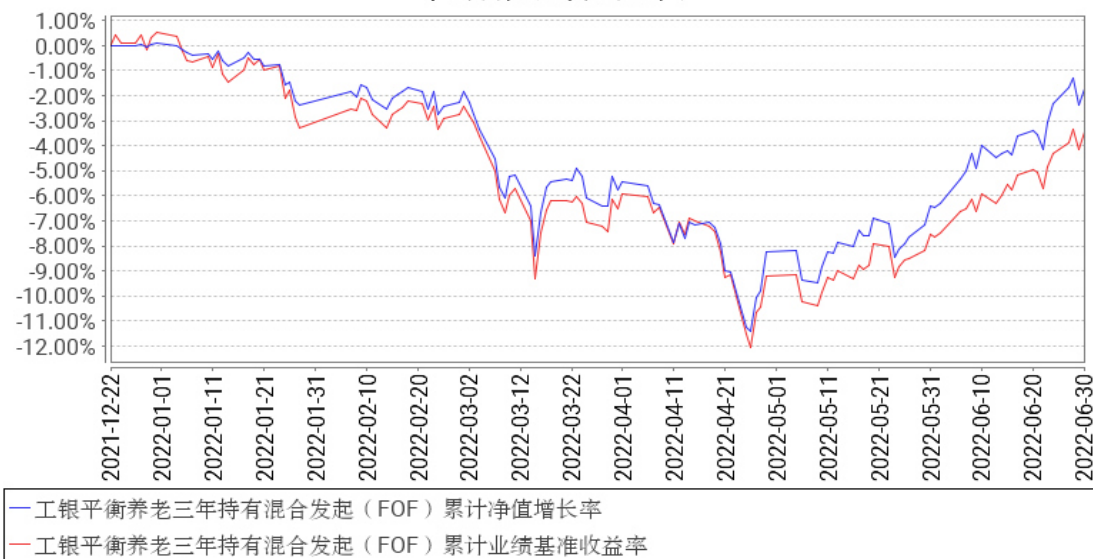
工银平衡养老三年持有混合发起（FOF）累计净值增长率与同期业绩比较基准收益率的历史走势对比图
