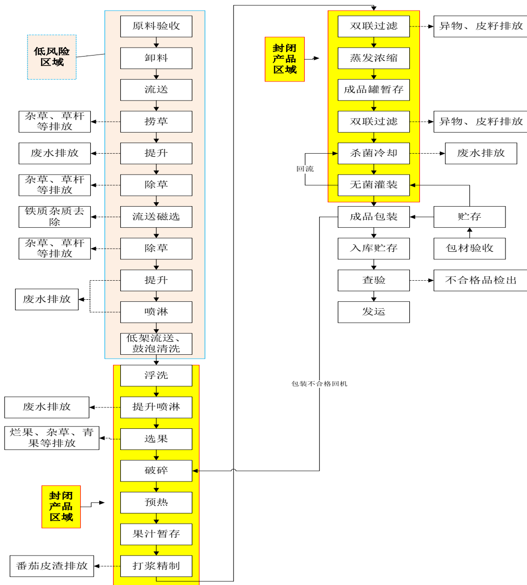
无菌袋装番茄酱工艺流程图
