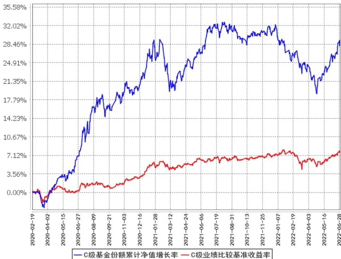
C级基金份额累计净值增长率与同期业绩比较基准收益率的历史走势对比图 (2020年2月19日至2022年6月30日)
