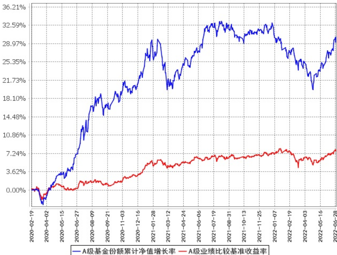
A级基金份额累计净值增长率与同期业绩比较基准收益率的历史走势对比图 (2020年2月19日至2022年6月30日)
