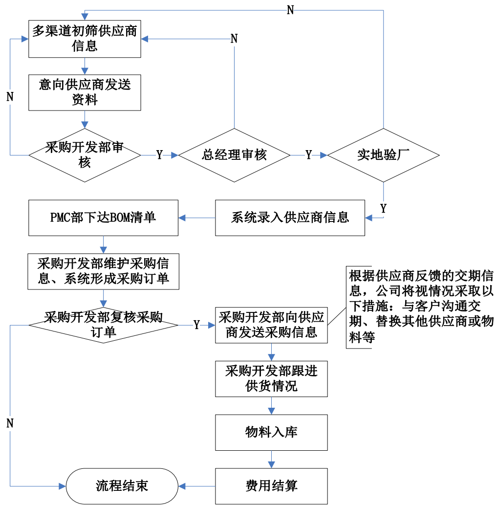
(2) 原材料入库及检验流程
