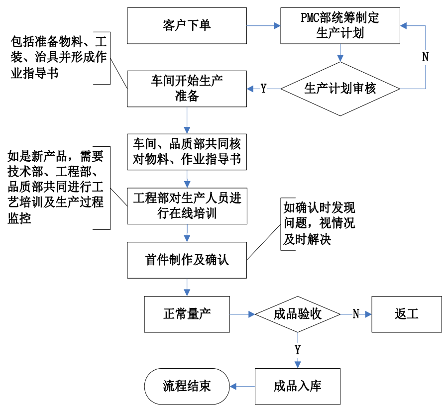
(2) PCBA 的生产工艺流程
