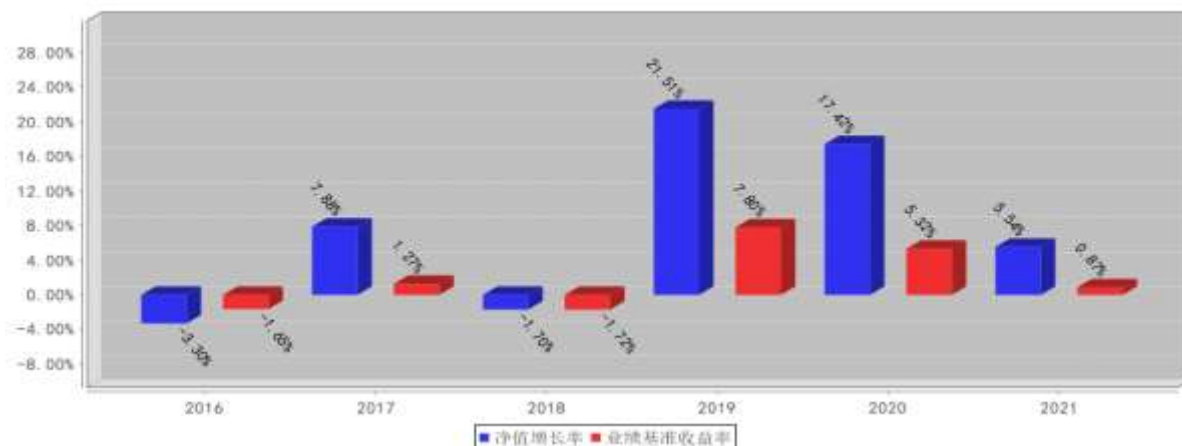
东方红价值精选混合C 基金每年净值增长率与同期业绩比较基准收益率的对比图（2021年12月31日）
