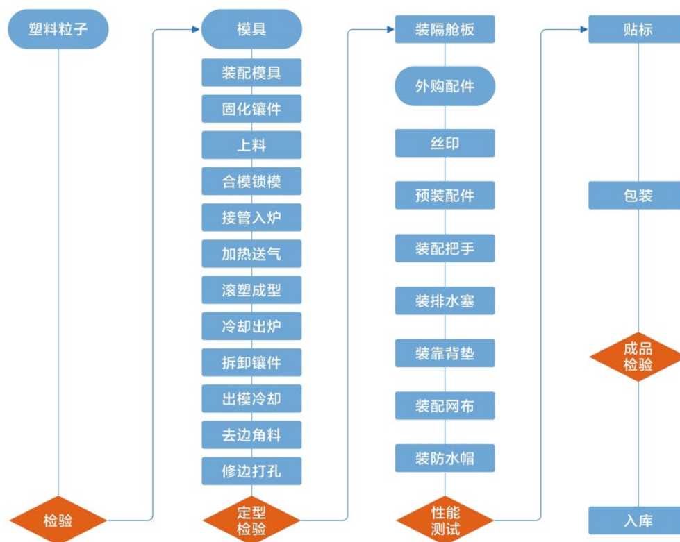
滚塑皮划艇生产工艺流程
