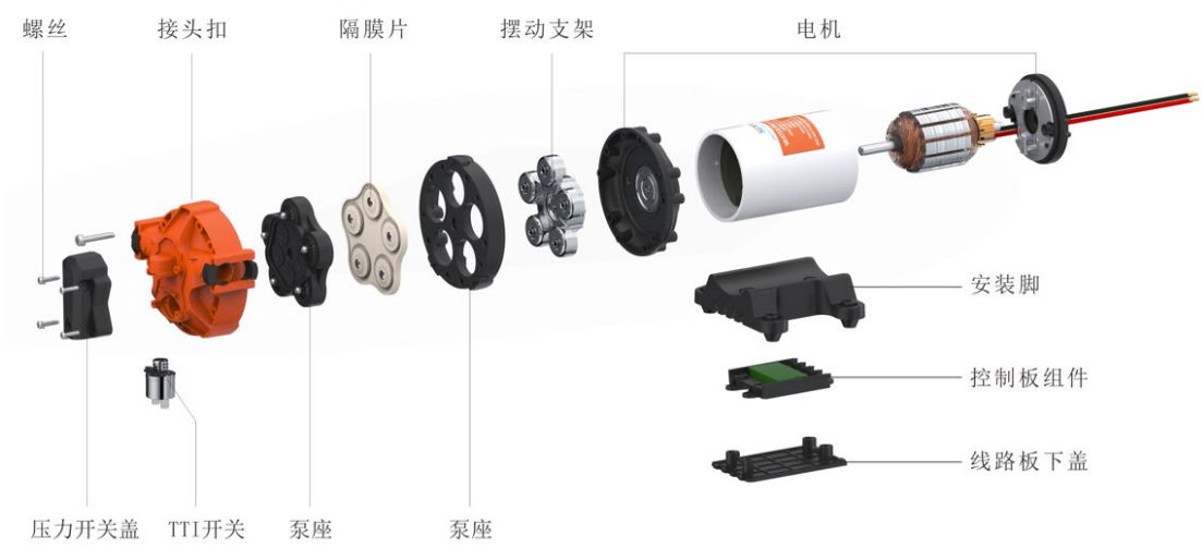
水泵结构图
