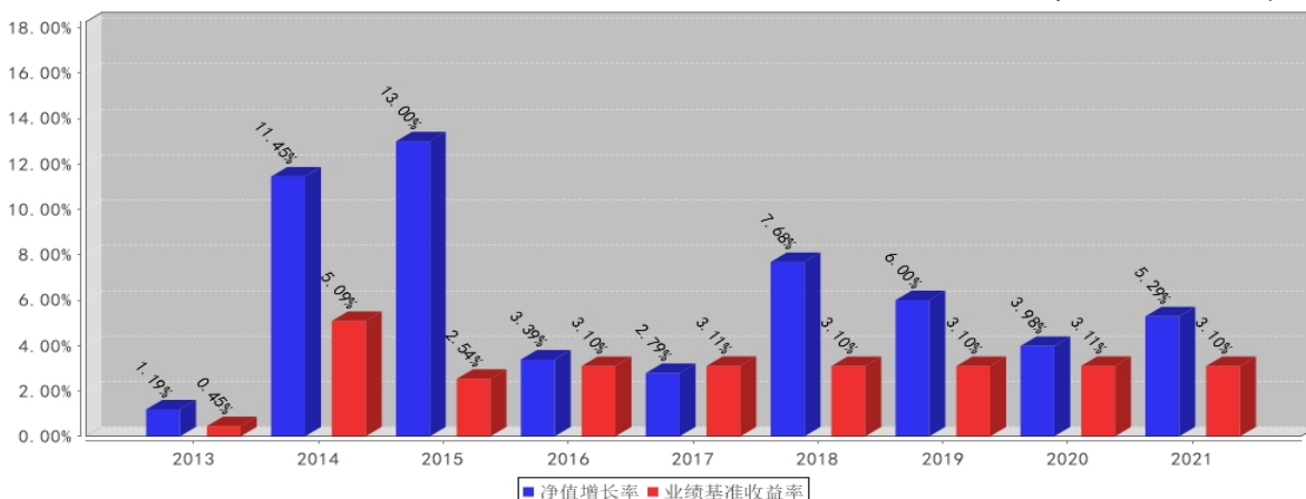
长信纯债一年定开债券A基金每年净值增长率与同期业绩比较基准收益率的对比图（2021年12月31日）
