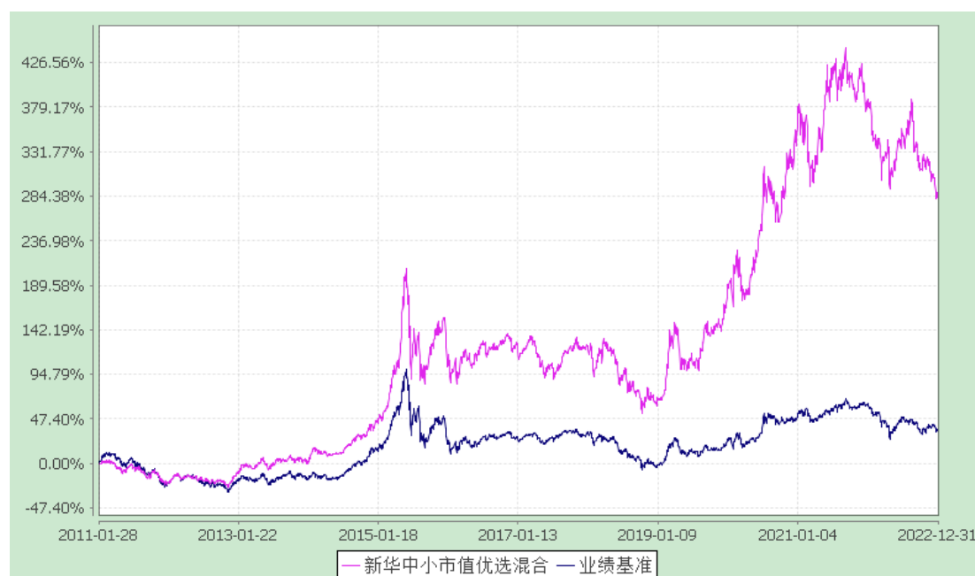
新华中小市值优选混合型证券投资基金 累计净值增长率与业绩比较基准收益率历史走势对比图 (2011 年 1 月 28 日至 2022 年 12 月 31 日)
