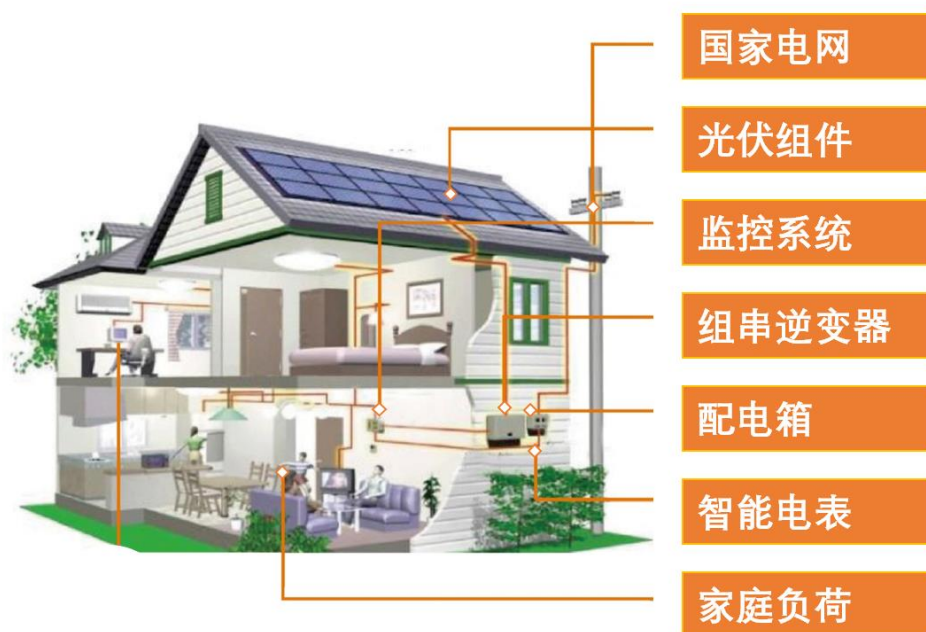
户用分布式光伏电站示例
