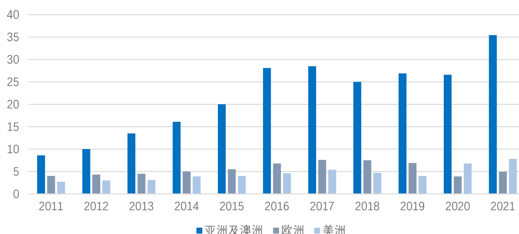
工业机器人年度安装总量(万台)
