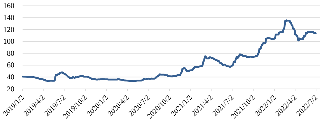
2019年1月-2022年6月镨钕市场价格走势（万元/吨）
