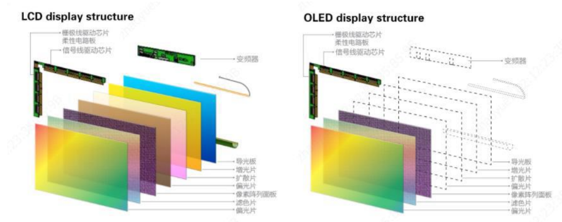
TFT-LCD 与 OLED 结构对比图
