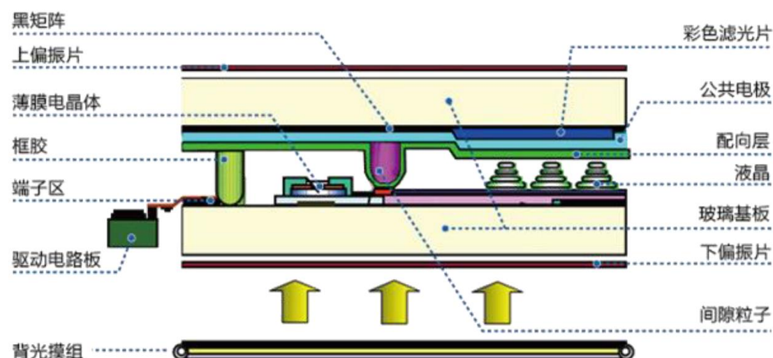
TFT-LCD 结构图
