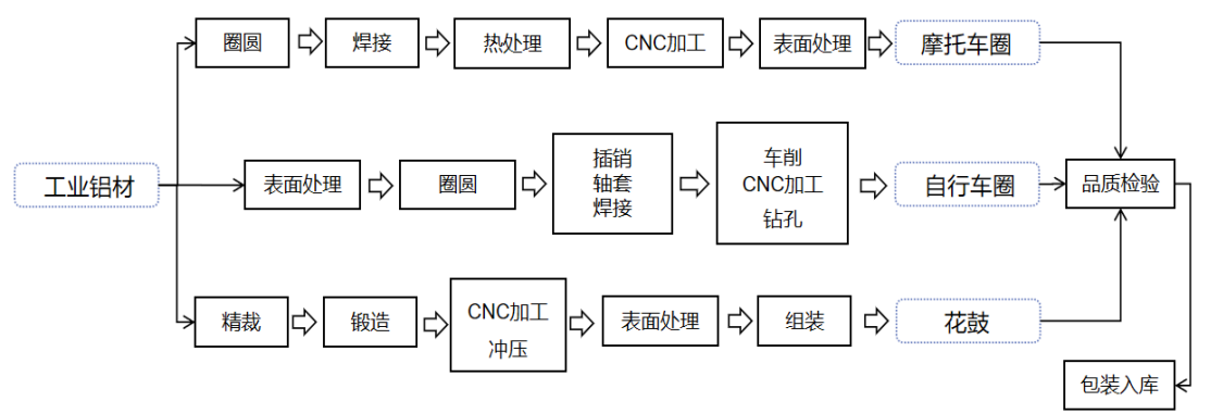
图：自行车及摩托车零部件工艺流程
