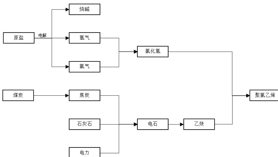
聚氯乙烯制造工艺示意图
