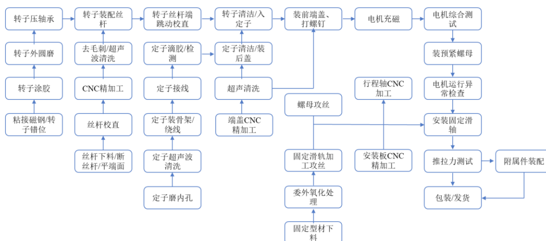
混合式步进电机生产流程图
