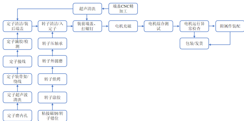
直流有槽电机生产流程图
