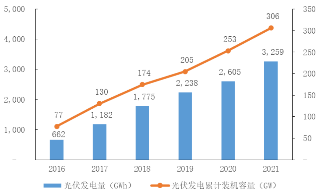
2016-2021 年我国光伏发电量与光伏发电累计装机量
