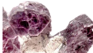
锂云母
