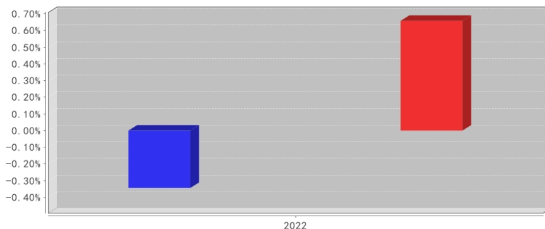
长信颐天养老三年持有混合（FOF）Y基金每年净值增长率与同期业绩比较基准收益率的对比图
