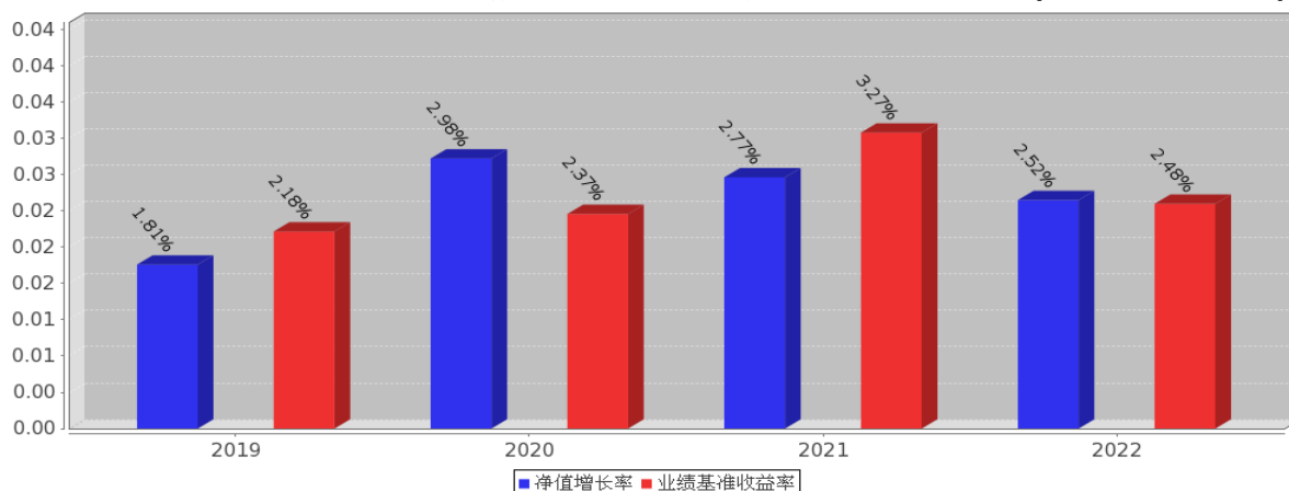
嘉实汇达中短债债券C基金每年净值增长率与同期业绩比较基准收益率的对比图(2022年12月31日)
