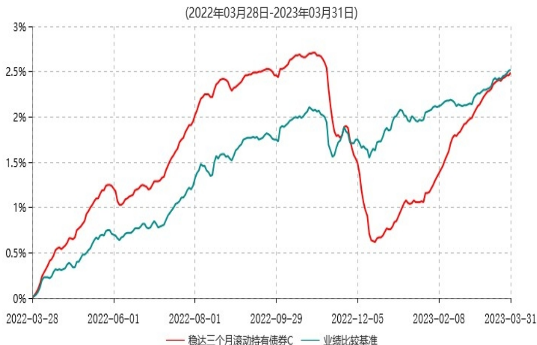
稳达三个月滚动持有债券C累计净值增长率与业绩比较基准收益率历史走势对比图
