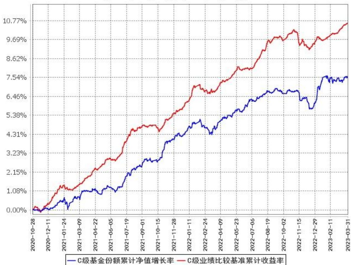
C级基金份额累计净值增长率与同期业绩比较基准收益率的历史走势对比图 (2020年10月28日至2023年3月31日)
