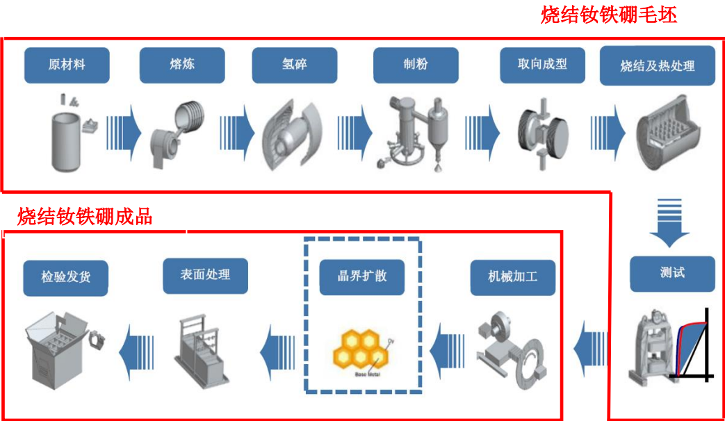
烧结钕铁硼生产工艺流程
