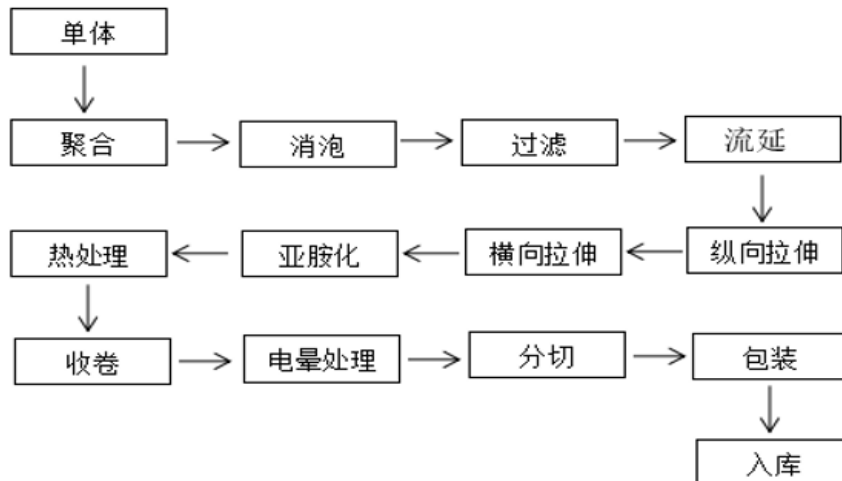
(4) 双轴定向法制膜生产流程图
