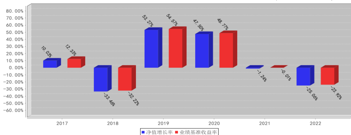
融通深证100指数C基金每年净值增长率与同期业绩比较基准收益率的对比图 (2022年12月31日)
