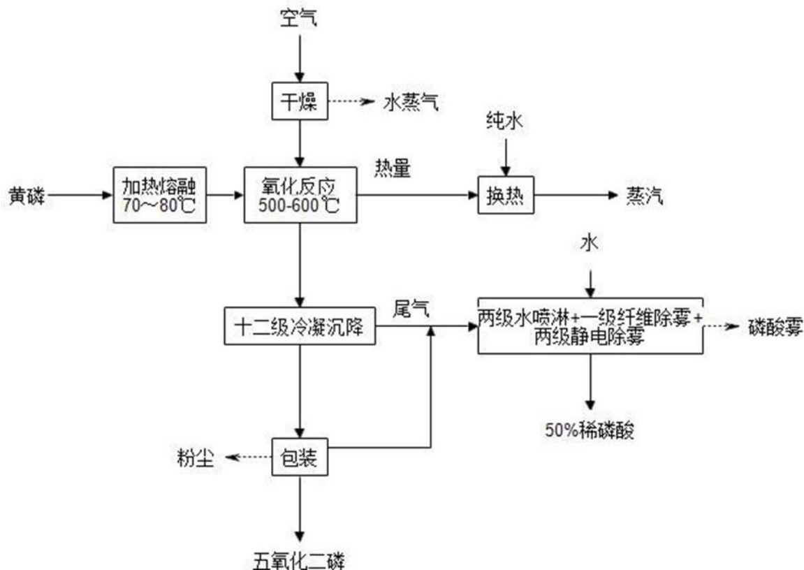
（1）五氧化二磷生产流程图及主要工艺说明
