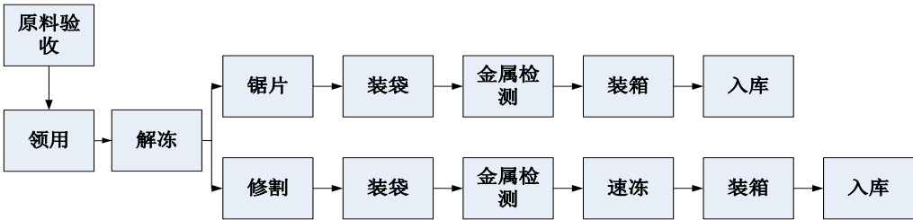
图 5-6 肉制品初加工工艺流程
