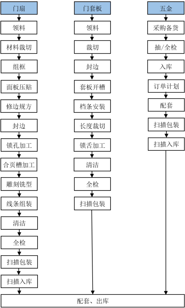
图 5-8 室内木门工艺流程图
