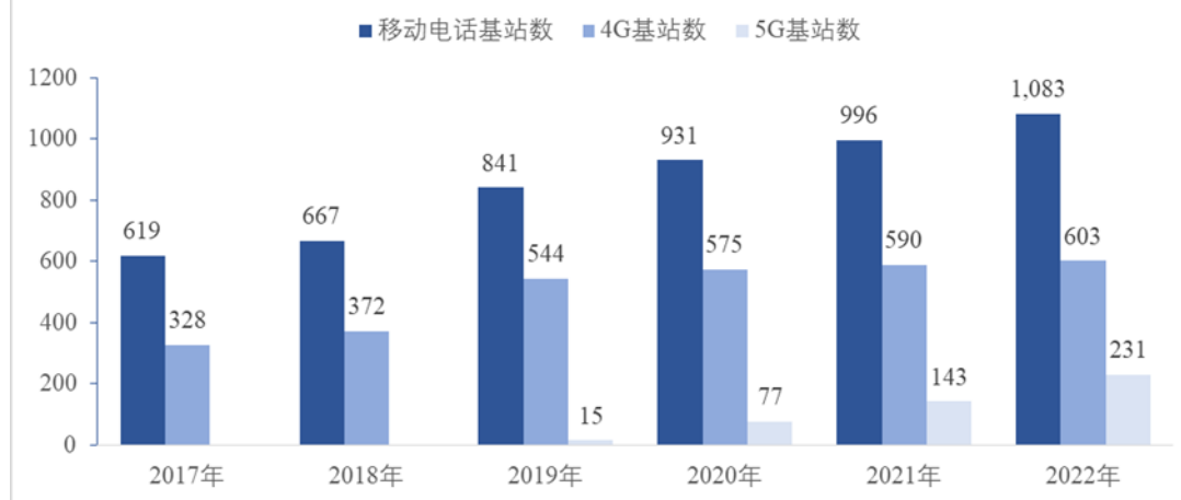
2017-2022年各类基站数量（单位：万个）
