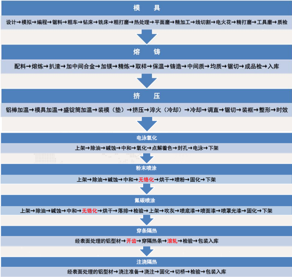
图：广亚铝业主要生产工艺流程图
