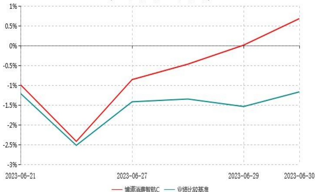
博道消费智航C累计净值增长率与业绩比较基准收益率历史走势对比图
