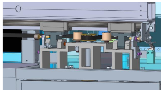
半高屏蔽门驱动系统
