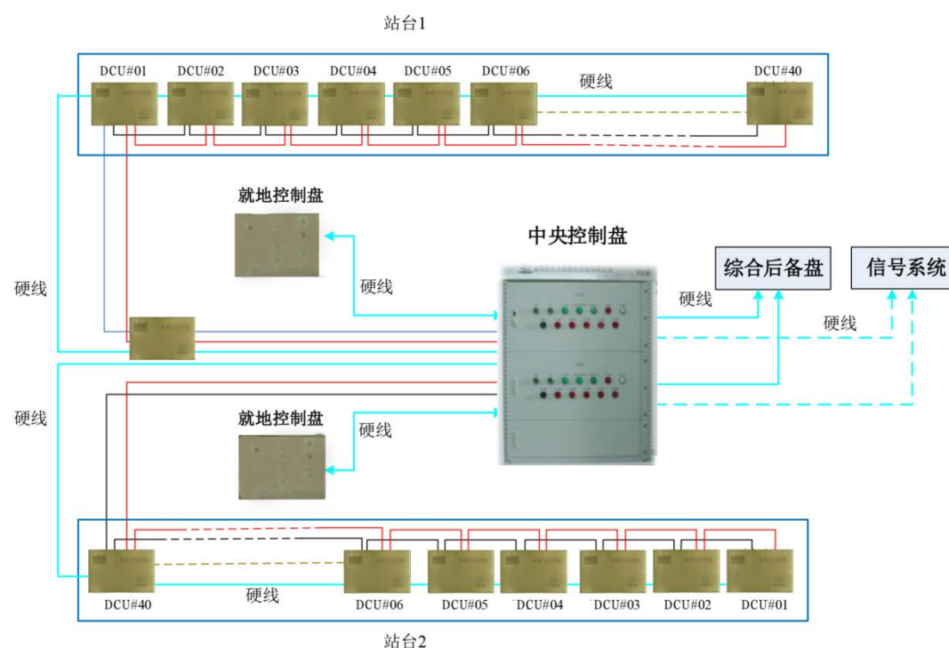
站台屏蔽门控制系统示意图
