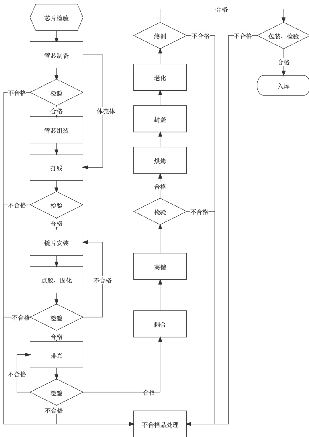
(2) 光纤激光器工艺流程图
