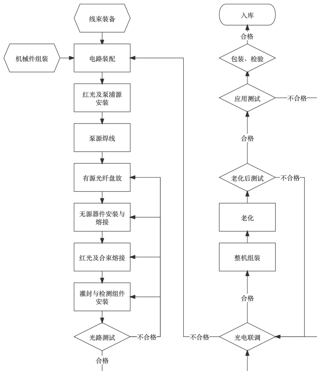
(3) 超快激光器系统工艺流程图
