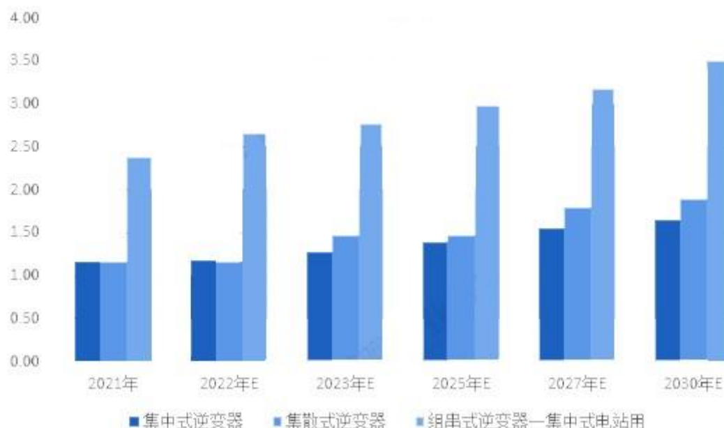
2021-2030年中国光伏逆变器功率密度变化趋势(单位: kW/kg)
