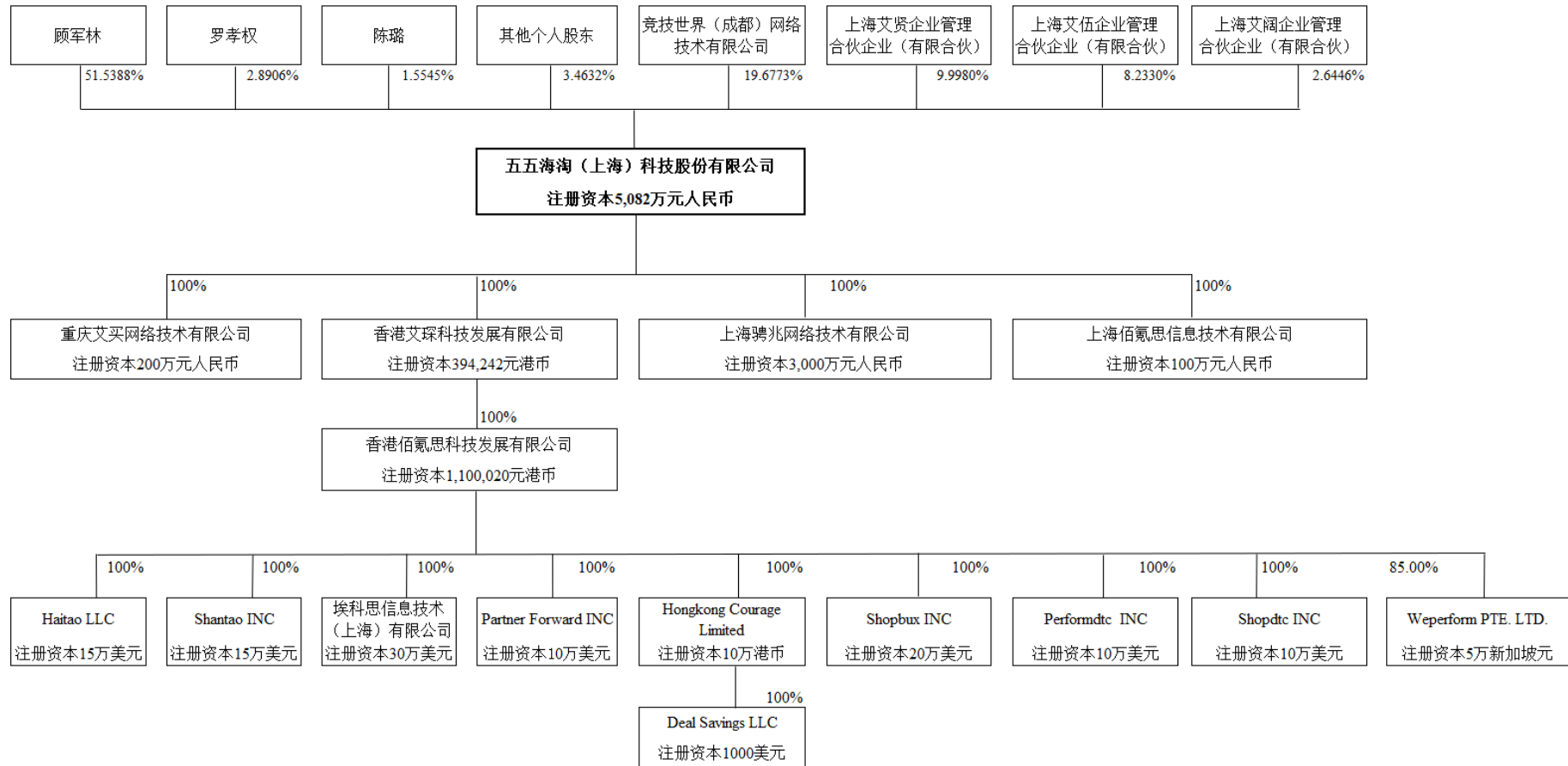
股权架构图
