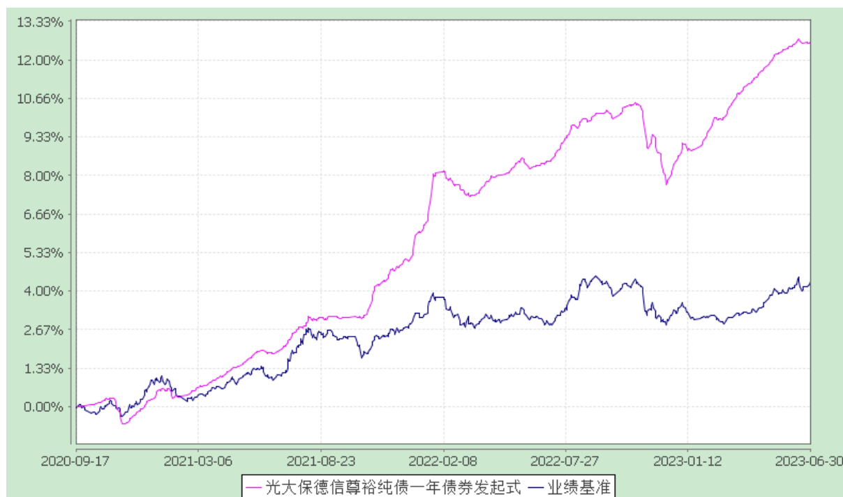
光大保德信尊裕纯债一年定期开放债券型发起式证券投资基金 份额累计净值增长率与业绩比较基准收益率历史走势对比图 (2020 年 9 月 17 日至 2023 年 6 月 30 日)
